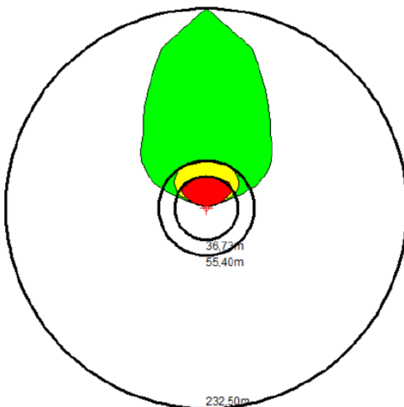
Slika 26: Prikaz rezultata modeliranja disperzije zapaljivih/eksplozivnih para benzina uslijed istjecanja medija iz autocisterne kapaciteta os 38.000 l
